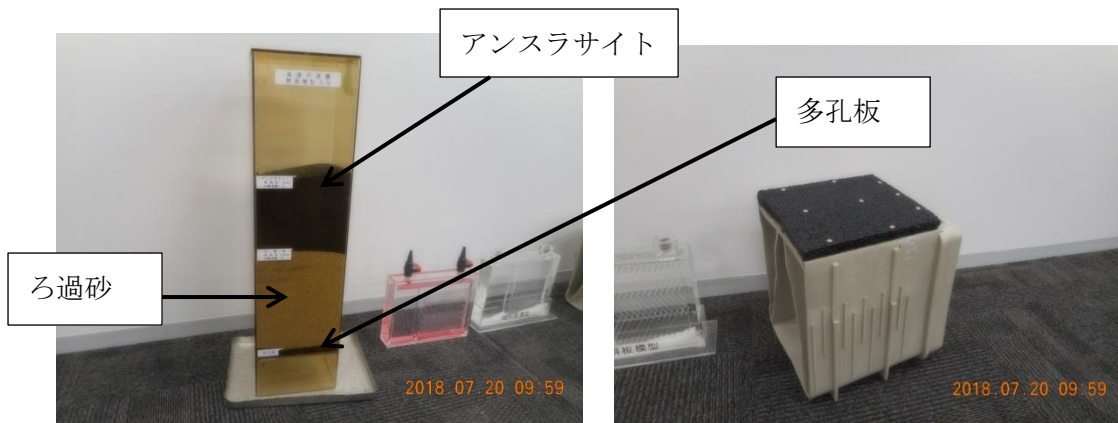
ろ過装置…アンストラサイト（無煙炭）と砂の層を通して微細な浮遊物を取り除く （長沢浄水場のパンフレットより）
